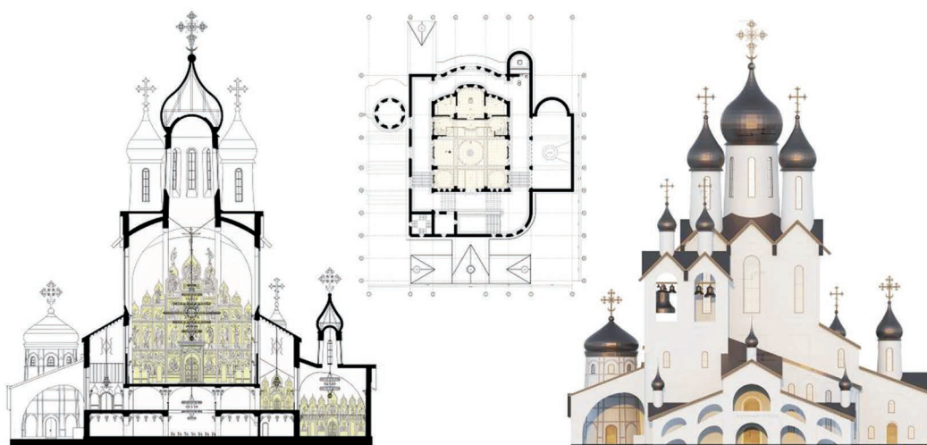
Рис. 5. Проект собора в с. Лопатино Ярославской области на реке Сить, автор Ф. В. Скисов
