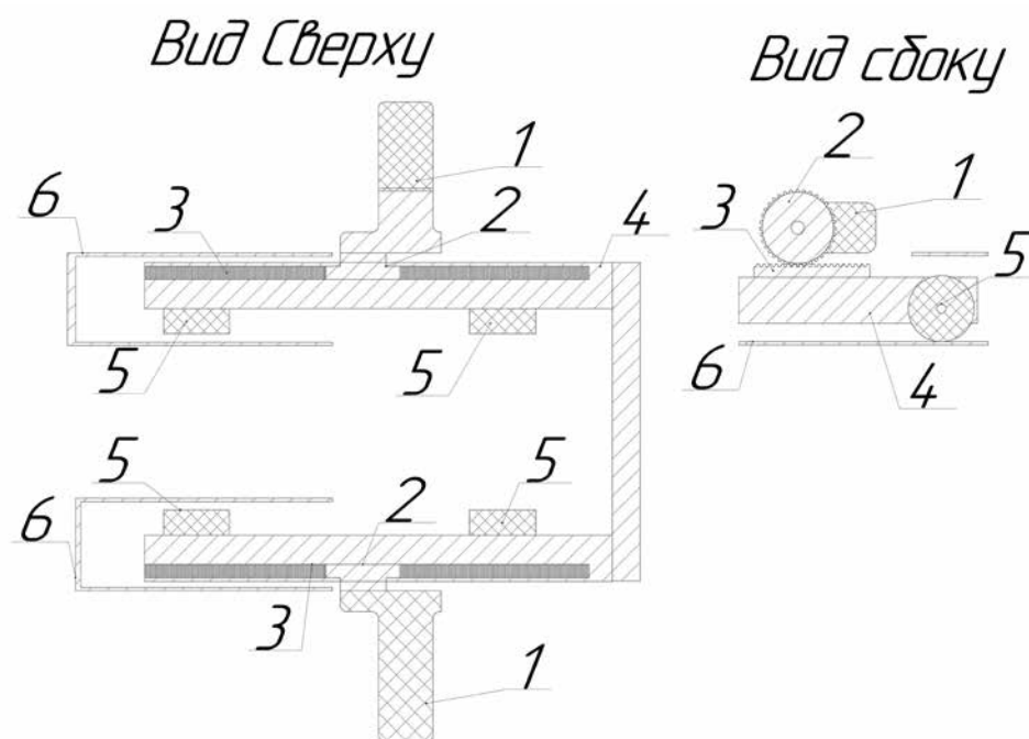
Рис. 1. Система slide out
